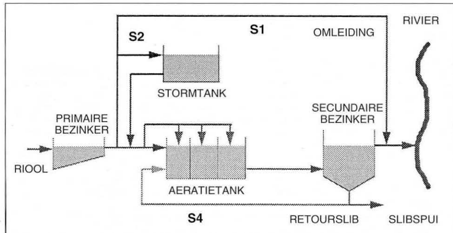
Fig. 1 Schematische weergave van het zuiveringsstation
