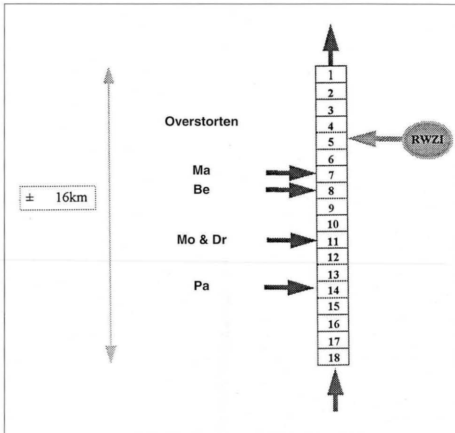
Fig. 2 Schematische voorstelling van het riviermodel
