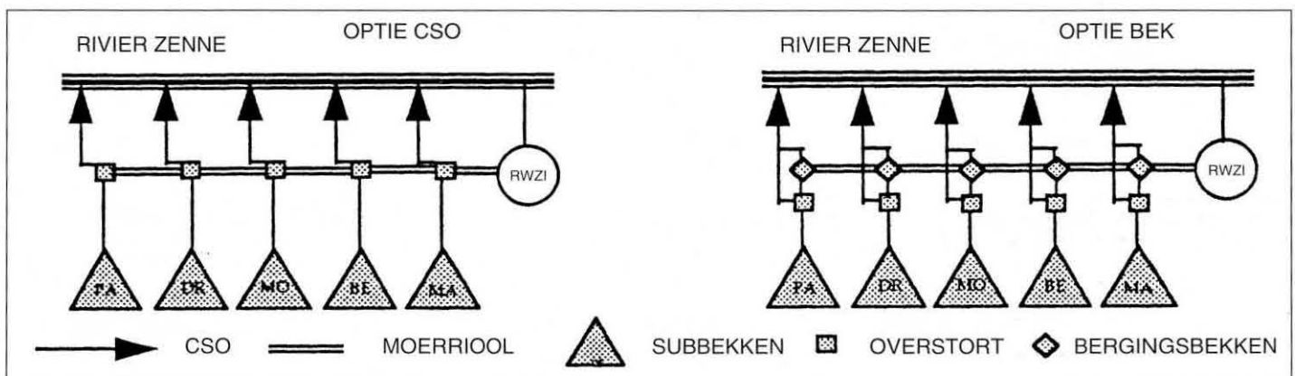
Fig.3 Het vereenvoudigd rioleringsstelsel voor de CSO en BEK opties
